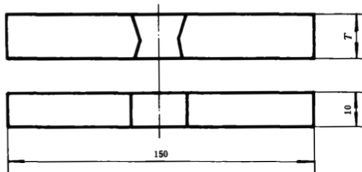
Hình A.4 – Mẫu thử uốn cạnh
