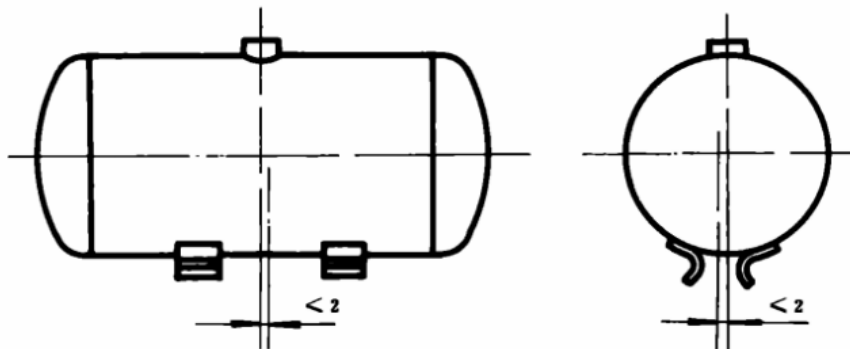
Hình 8 – Đường trung tâm ngang, dọc
