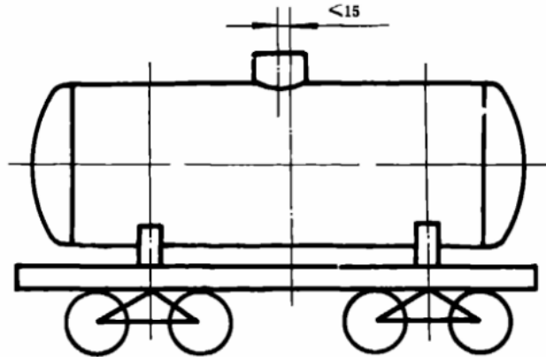
Hình 11 – Sai lệch giữa trục dọc thân bồn và trục dọc bộ xe
