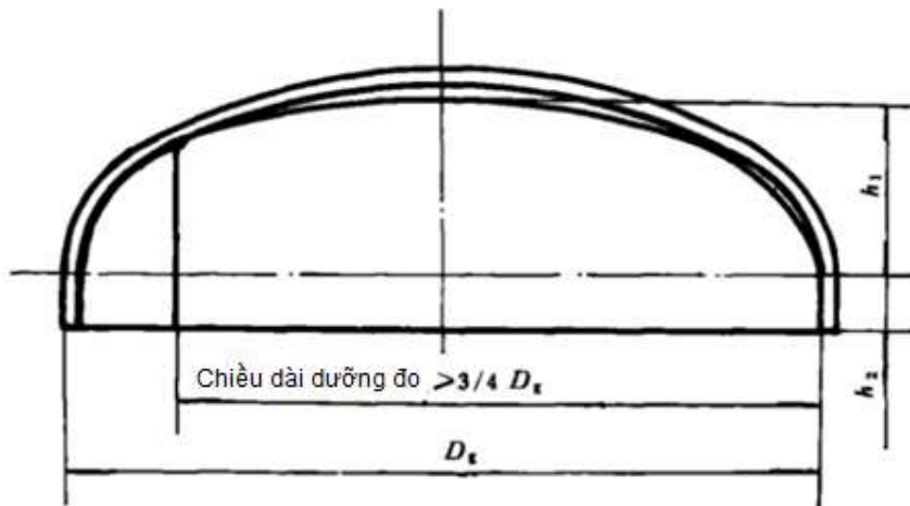
Hình 2 – Kích thước nắp đầu bồn xi téc
