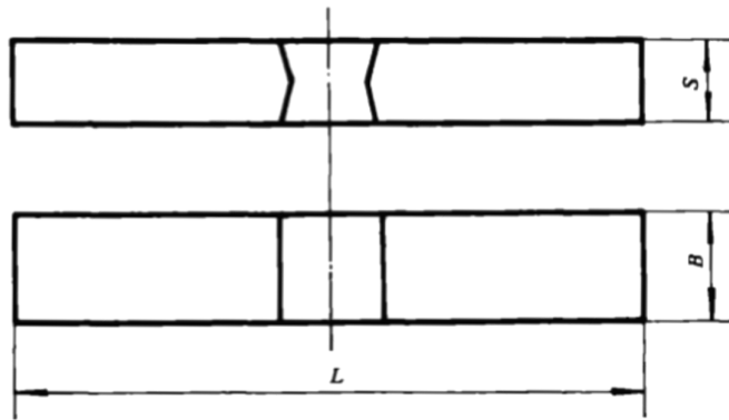
Hình A.3 – Mẫu thử uốn ngang
