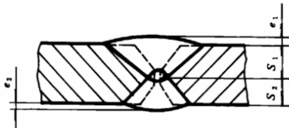
Hình 9 – Mối hàn giáp mép
