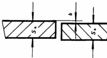
Hình 6 – Kích thước sai lệch giáp mối
