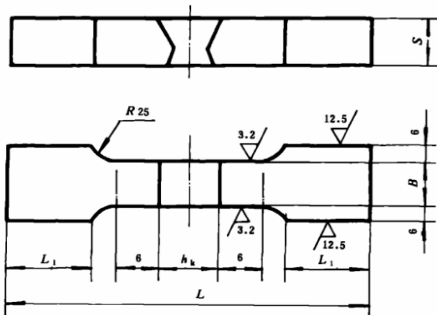
Hình A.2 – Mẫu thử kéo
