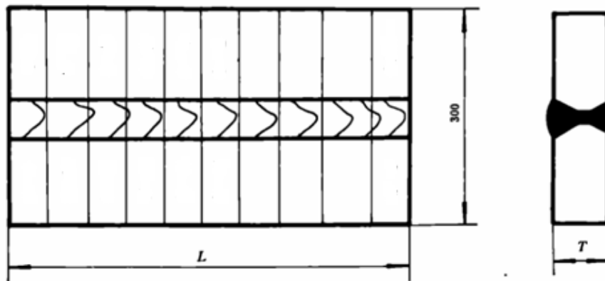
Hình A.1 – Kích thước tấm thử và lấy mẫu thử
