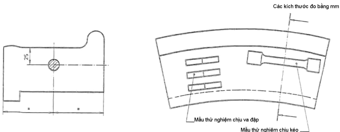
Hình 1 – Vị trí của các mẫu thử chịu kéo và va đập
