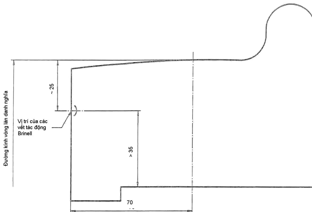
Hình 3 – Vị trí của các vết tác động độ cứng Brinell
