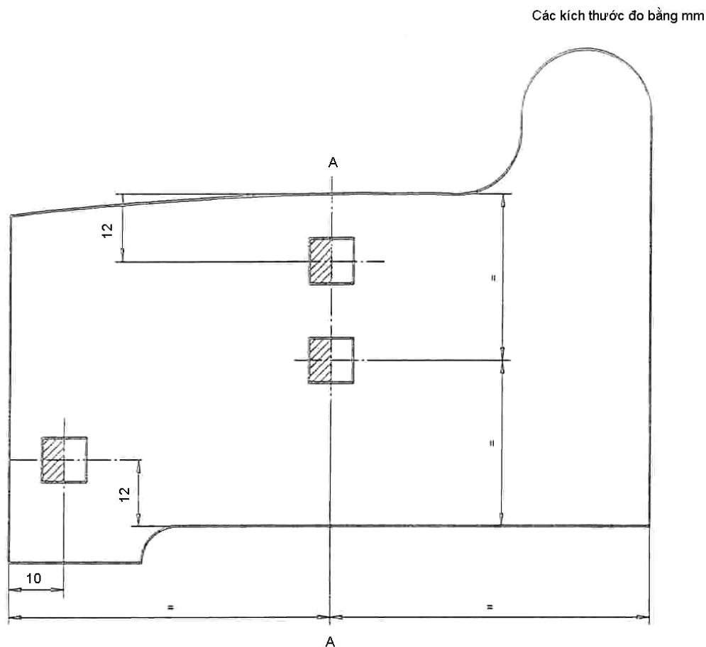
Hình 2 – Vị trí của mẫu thử va đập
