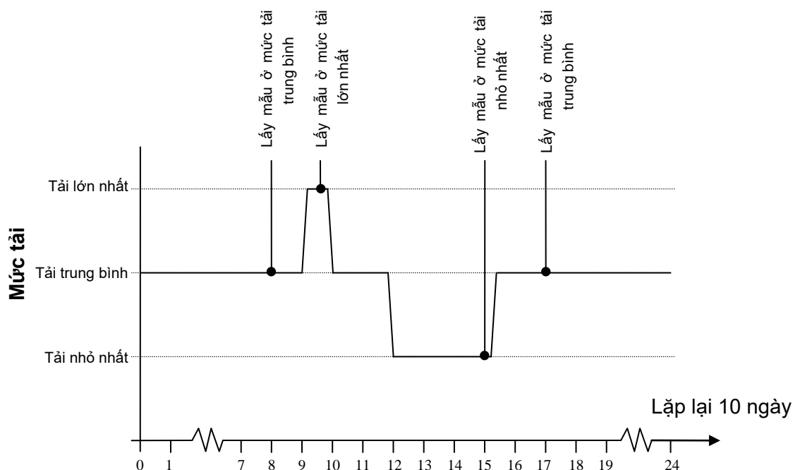
Hình 2. Các mức tải thủy lực đề nghị và tần suất lấy mẫu thử cho hệ thống xử lý nước thải (có thể được thay đổi nếu cần thiết khi xét đến các đặc điểm của mỗi hệ thống xử lý nước thải)
