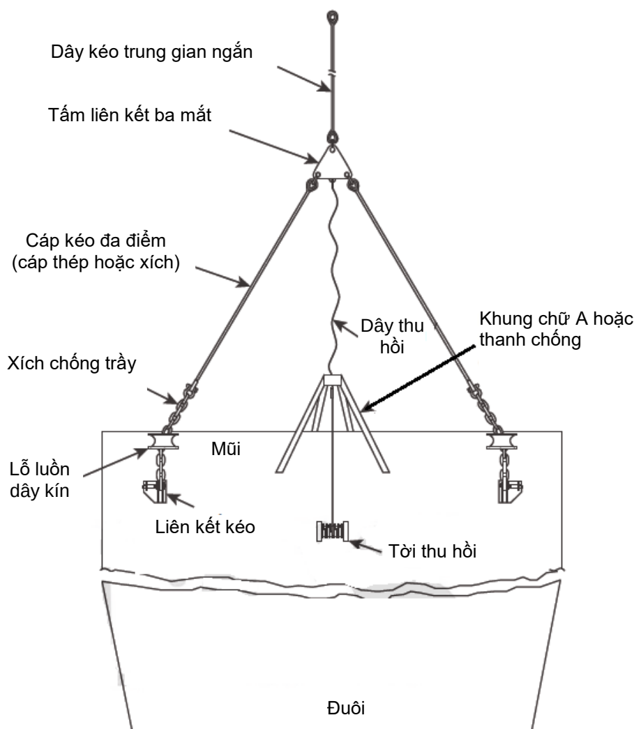
Hình 5.3.13 Bố trí hệ thống thu hồi cáp kéo đa điểm/xích kéo đa điểm
