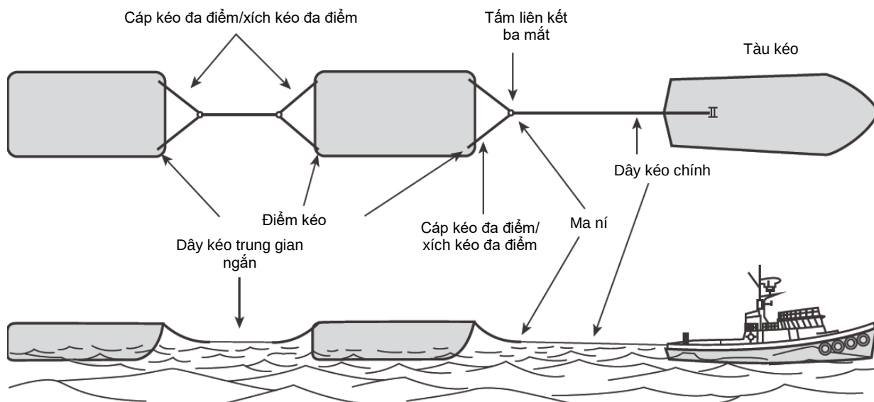
Hình 1.2 Sơ đồ bố trí kéo nối tiếp
