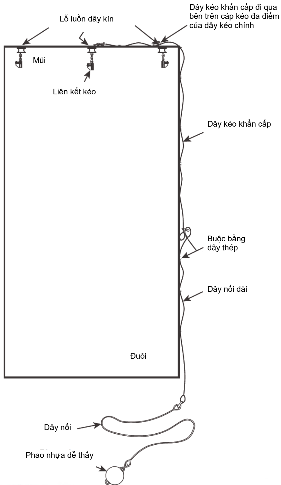
Hình 5.3.16 Bố trí dây kéo sự cố cố định trên đối tượng được kéo không có người trực
