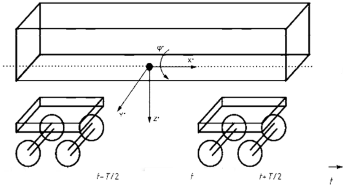
Hình A.1 – Hệ tọa độ địa phương đối với thân xe
