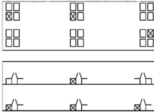
Hình 2 – Vị trí các điểm đo phương tiện 2 tầng (thông thường hoặc được ghép lại)
