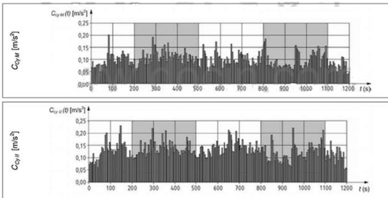
Hình D.1–Độ thoải mái liên tục–Tập hợp các khoảng thời gian 5 phút (các khoảng lựa chọn màu xám)
