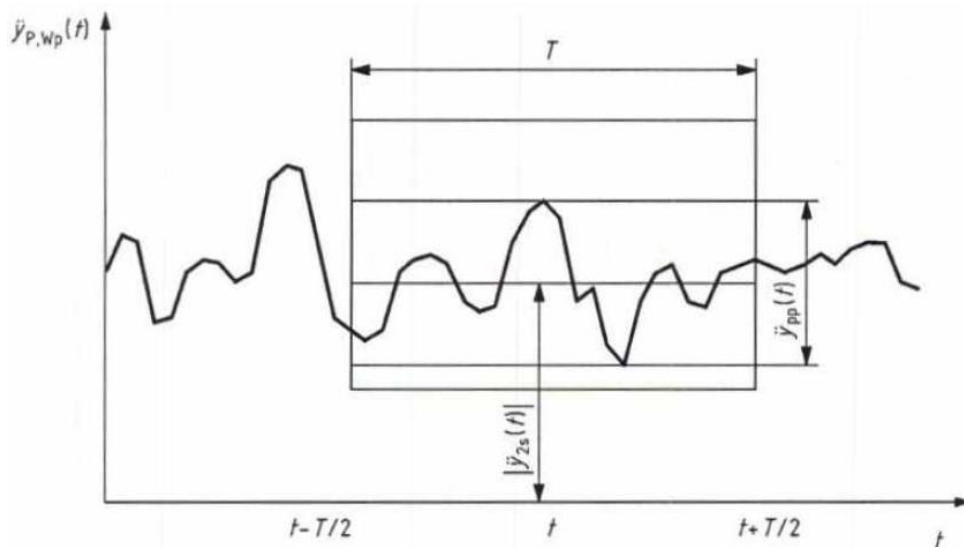
Hình 6 – Giải thích giá trị |\ddot{y}_{2s}^*(t)| và \ddot{y}_{pp}(t) để tính toán P_{DE}
