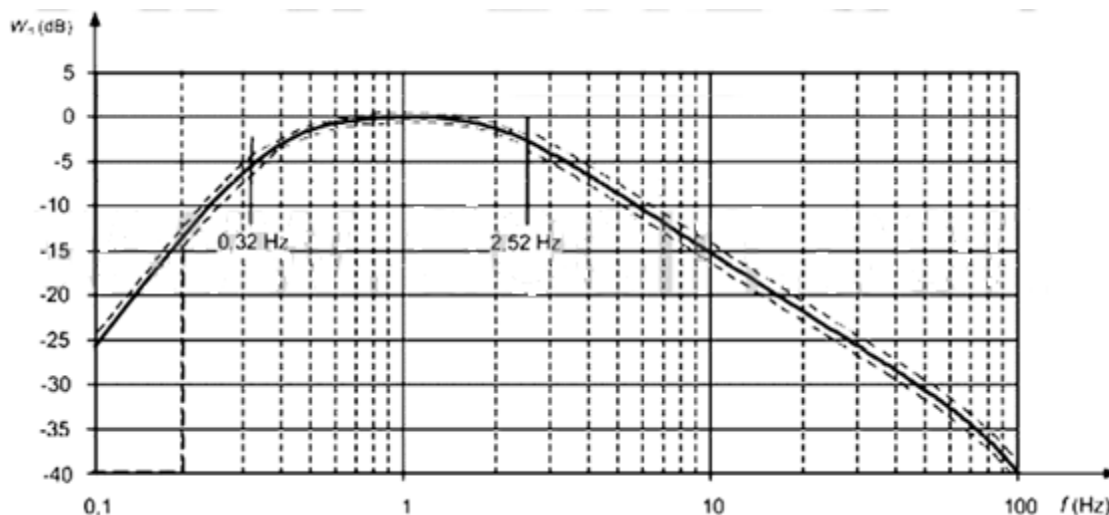
Hình C.7 – Biên độ của W_d trọng số tần số của rung động ngang dọc theo trục x hoặc y trên sàn xe, hoặc dọc theo trục y trên vải bọc ghế
