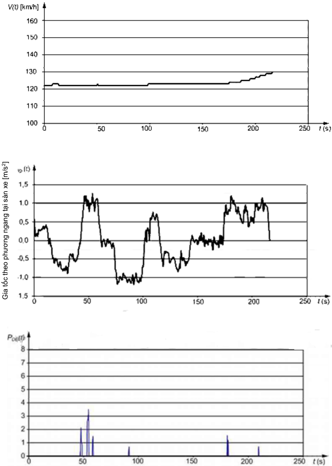
Hình D.4 – Ví dụ về biểu đồ thời gian đánh giá P_{DE}
