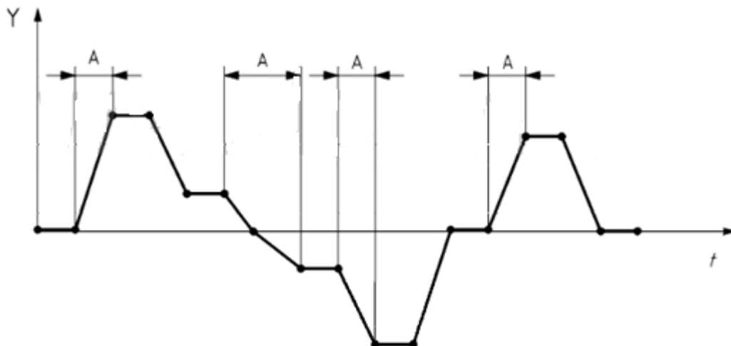
Hình 4 – Giải thích thuật ngữ |\dot{\varphi}_{1s}|_{\max} trong công thức P_{CT}
